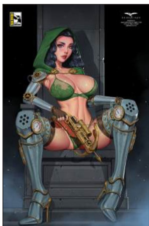
Dravacus - RHESJJ
